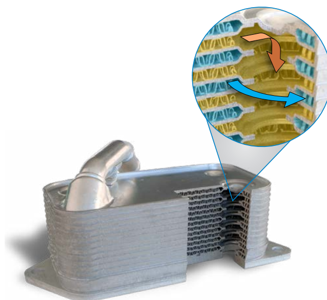
Масляный теплообменник для легкового автомобиля
