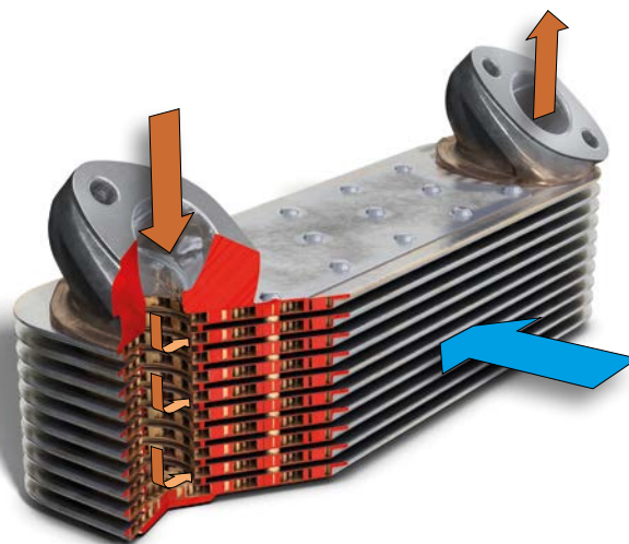
Масляный теплообменник для грузового автомобиля
